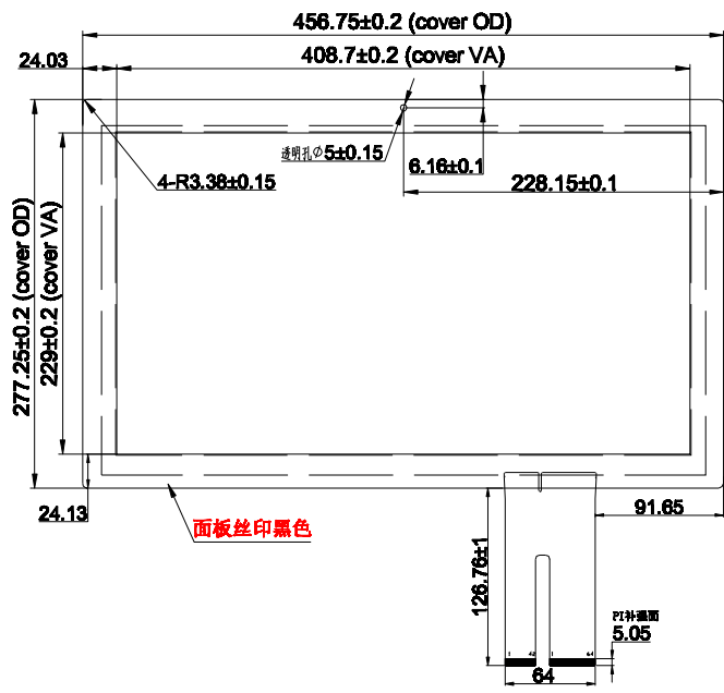
前视图 1:1
