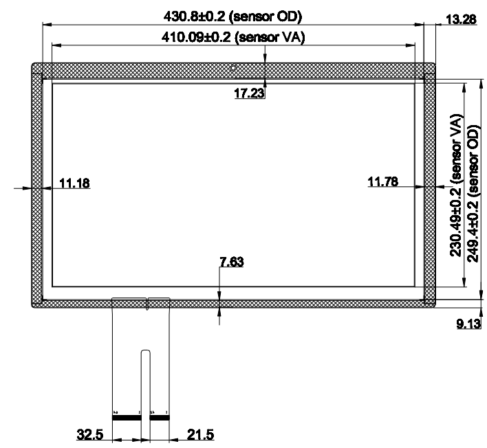
后视图 1:1
