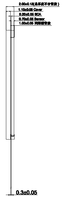
侧视图 横向10:1
